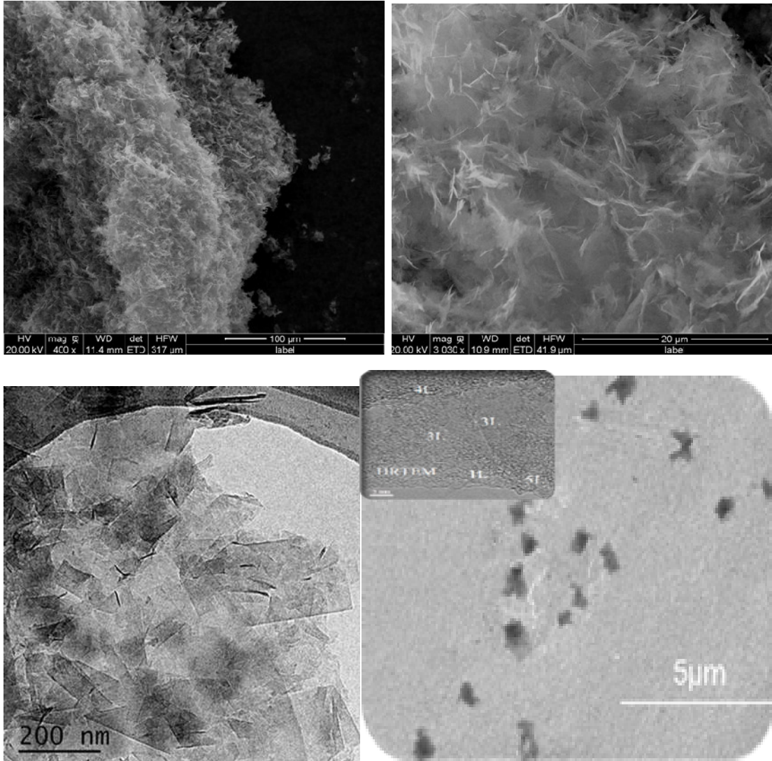
小尺寸薄层石墨烯扫描电镜、透射电镜分析图
